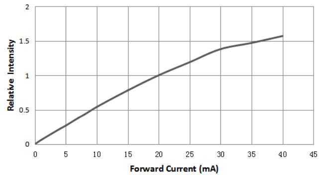
相对光强与电流特性曲线
