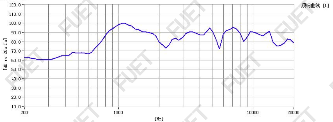
频响曲线
