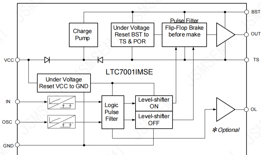
图 7-1 LTC7001IMSE功能框图
