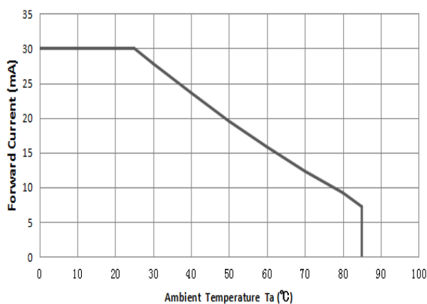
最大正向电流与环境温度特性曲线
