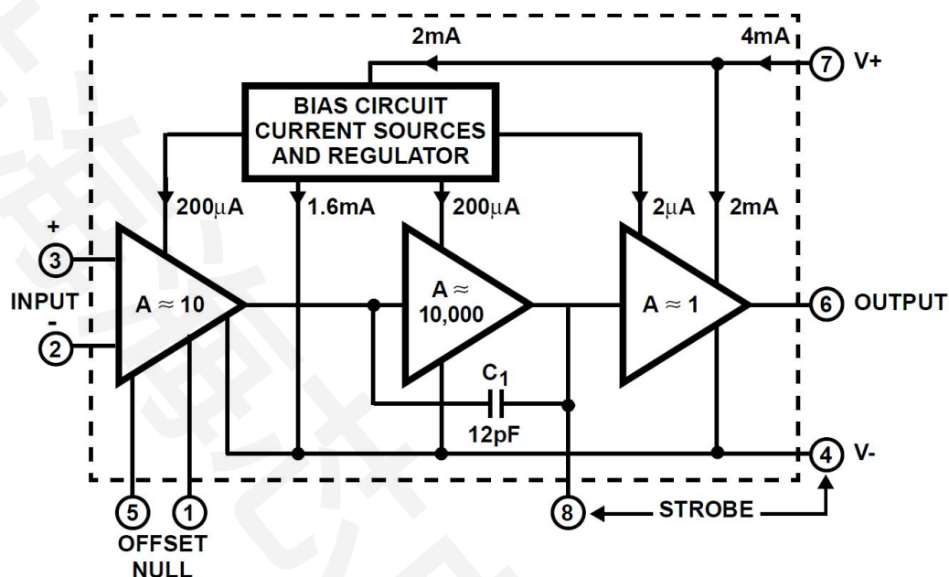
结构框图
