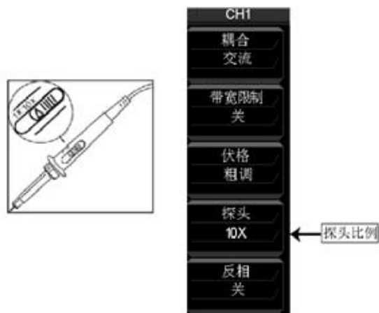
图1—5探头在数字存储示波器上的偏转系数设定
