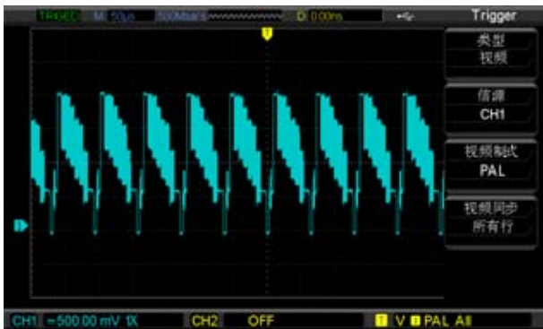
图2－16 视频触发：行同步
