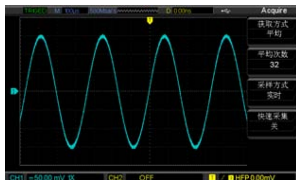
图2-21未采用平均的波形 图2-22采用32次平均的波形
