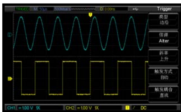
图2-18交替触发方式观察二个不同频率的信号
