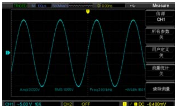
图 3-1 自动测量
