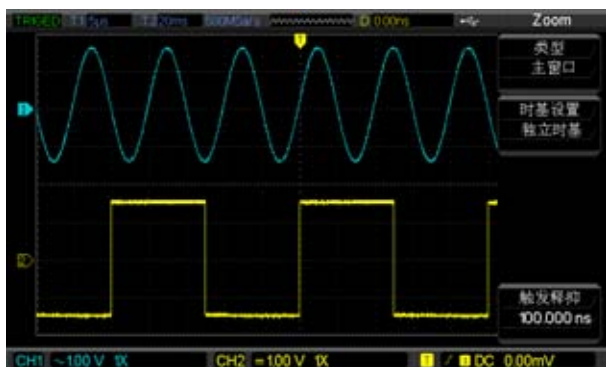
图2-14 独立时基同时显示两个频率不同的信号
