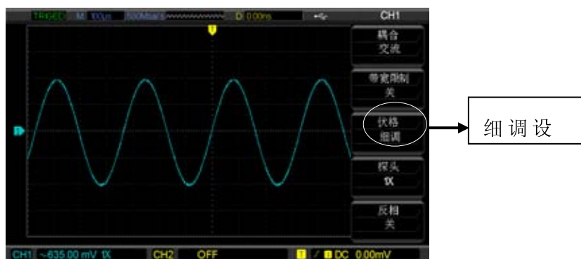
图2-7 垂直偏转系数粗调和细调
