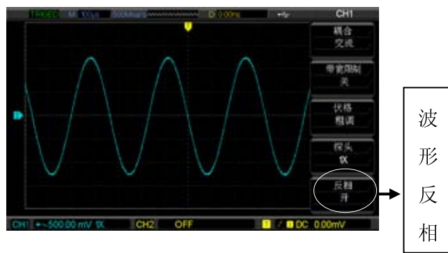
图2-9 垂直通道反相设置（反相）
