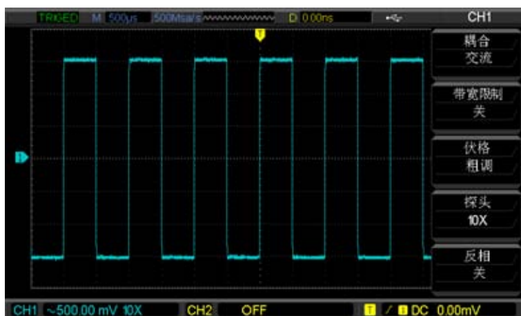
图1—6探头补偿信号
