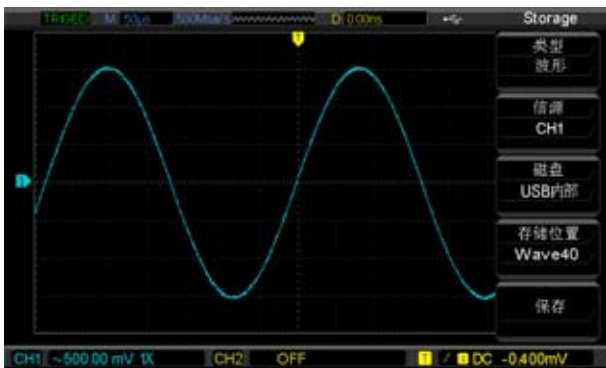
图2-26用U盘进行波形存储
