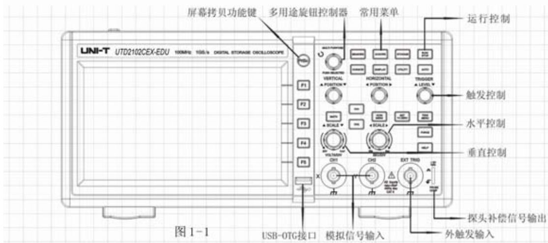
图 1-1 UTD2102CEX-EDU 前面板
