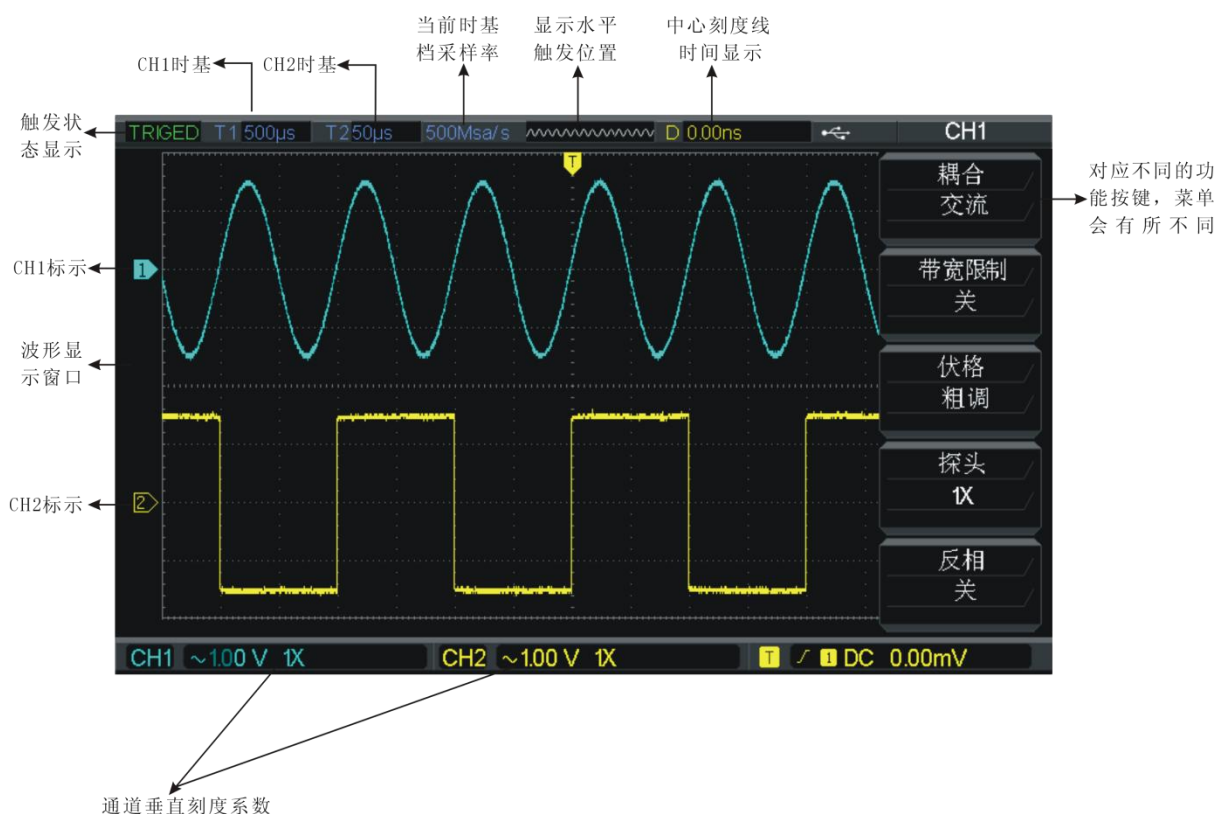
图1-2 UTD2102CEX-EDU数字存储示波器界面显示图
