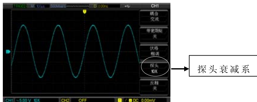
图2-6 通道菜单中的探头衰减系数设定
