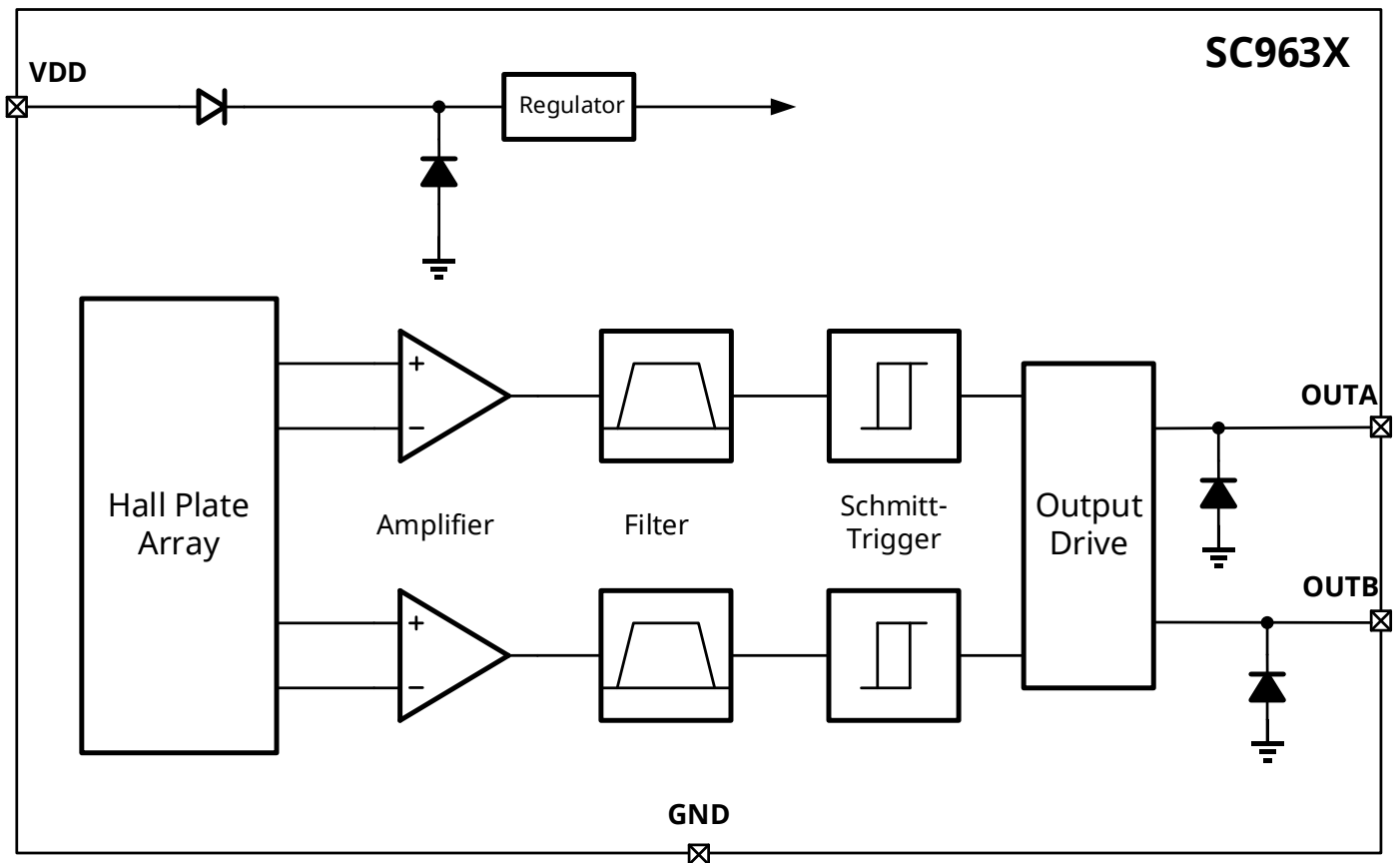
图 7 功能框图
