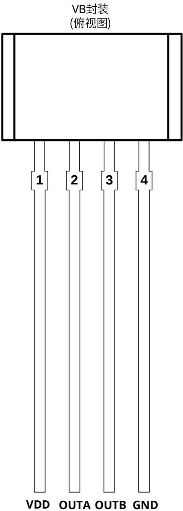
图 2 引脚描述
