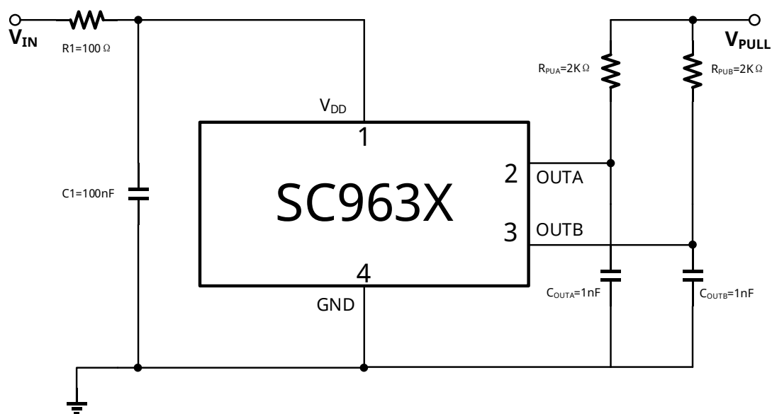
图 9 典型应用电路
