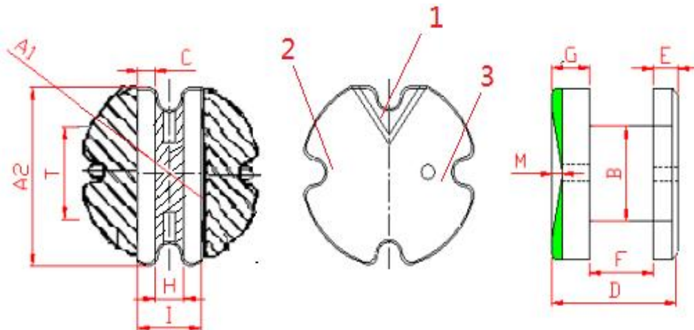
底部锡面图 (阴影区为锡面区)
