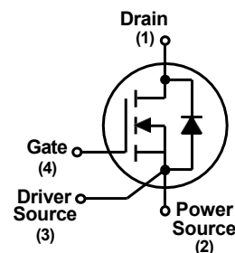
TO-247-4L
