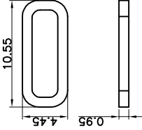
防水圈图示
