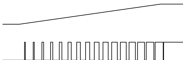
GP9303M与GP9303输出信号关系
