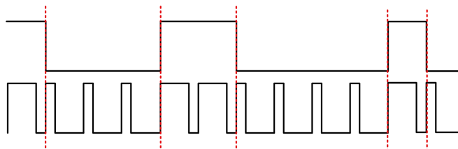
GP9303M与GP9303输出信号关系
