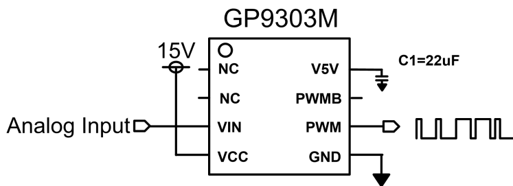
GP9303 电压转PWM关系
