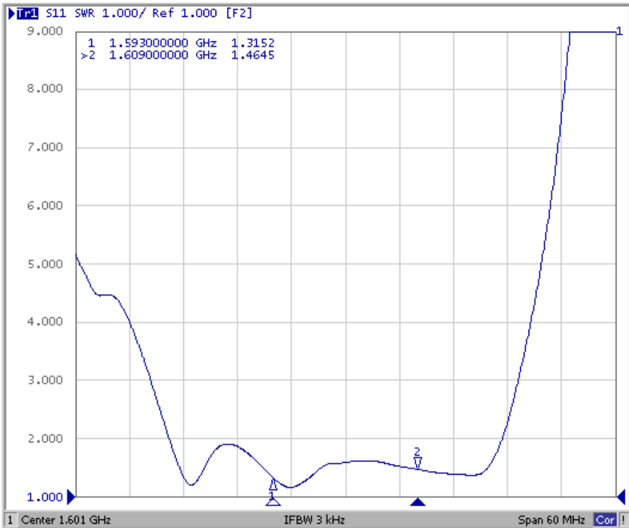
S11 VSWR
