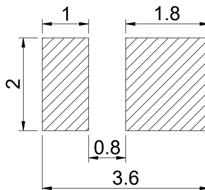
焊盘建议图
