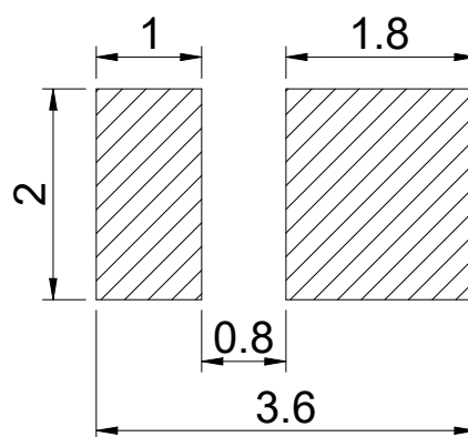
焊盘建议图
