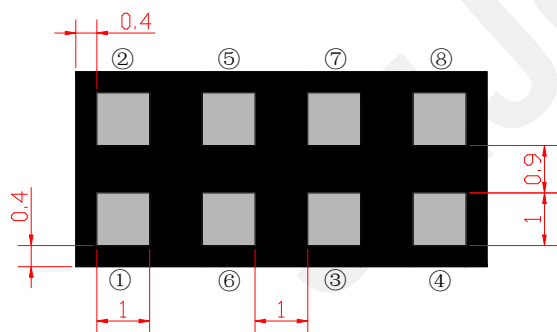
焊盘建议图
