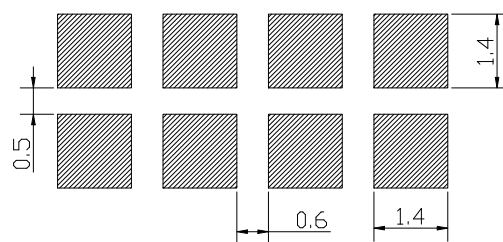
焊盘建议图
