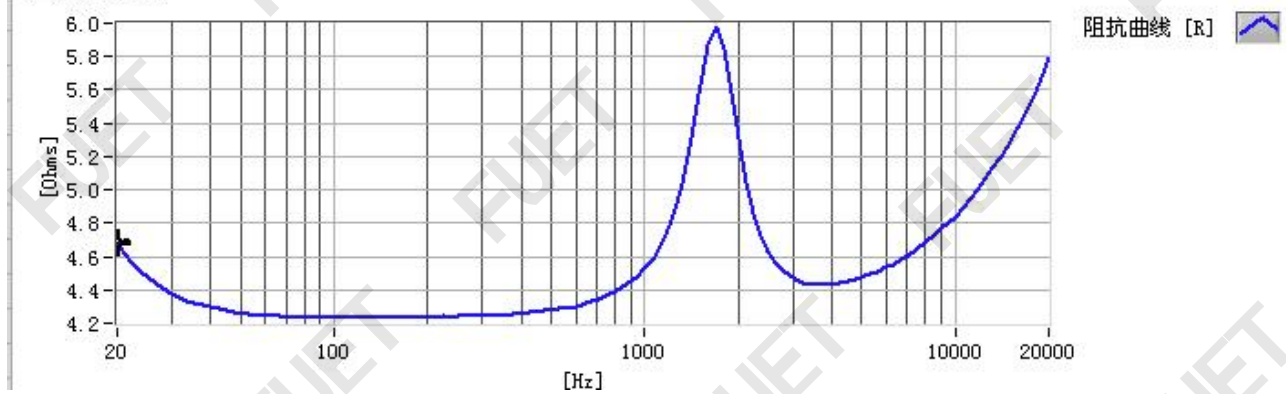
阻抗曲线
