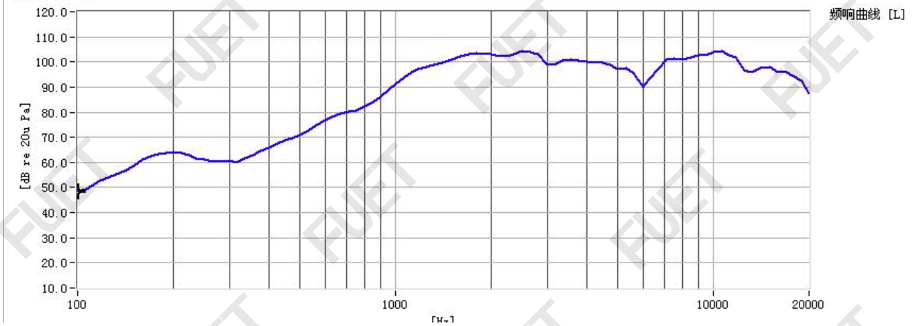
频响曲线
