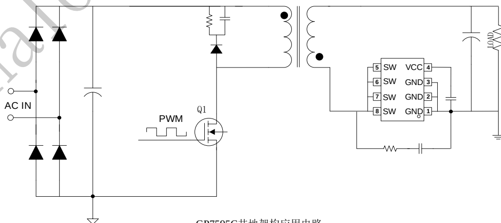
GP7595C共地架构应用电路
