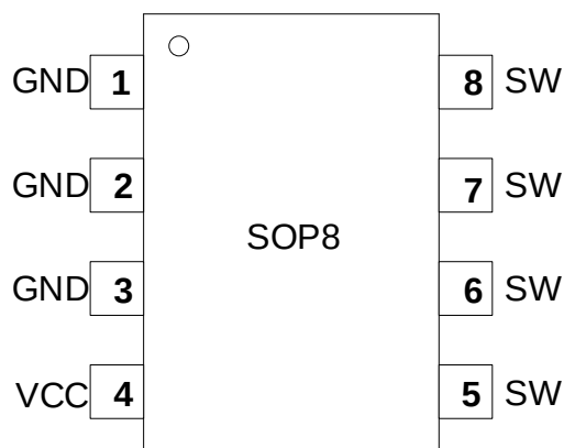
图 2 管脚封装图
