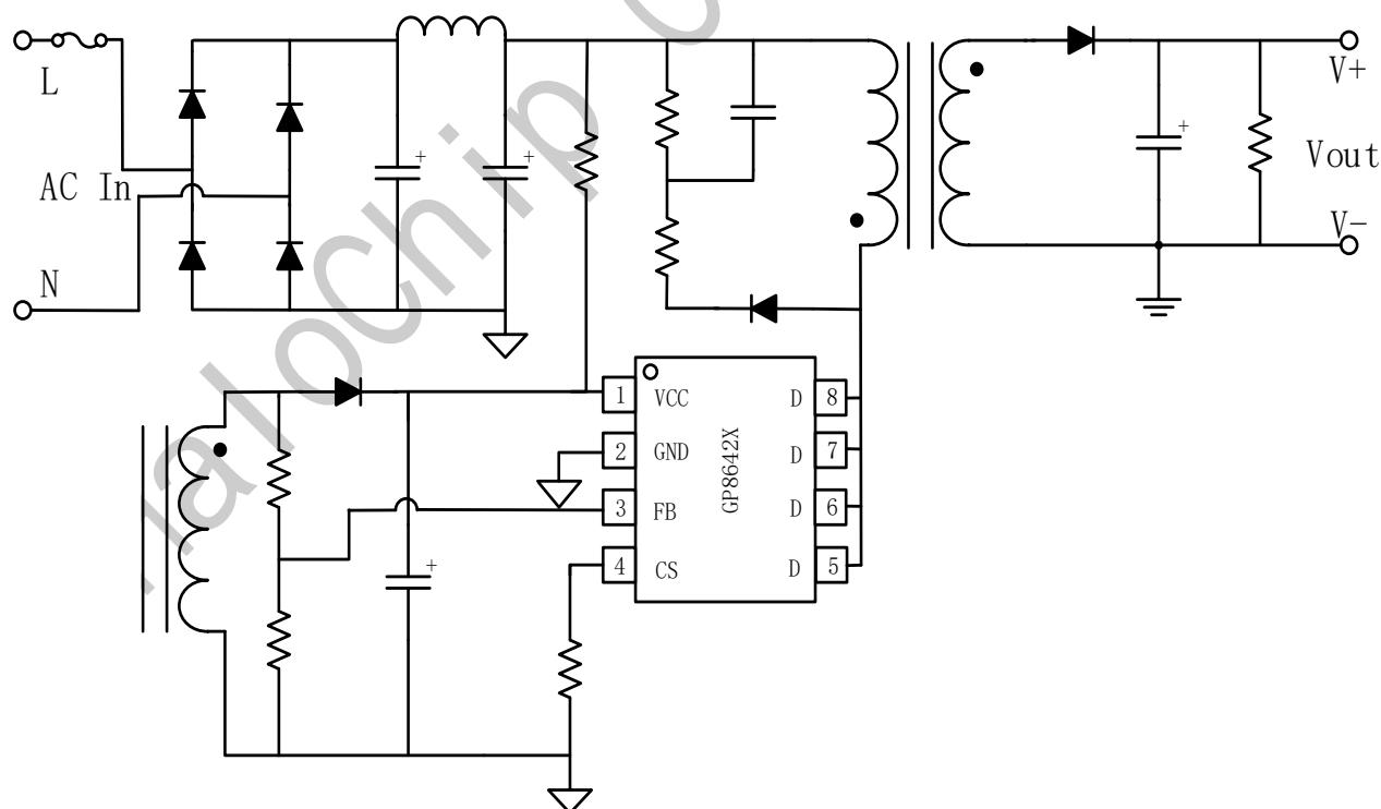
图 1 GP8642X 典型应用电路
