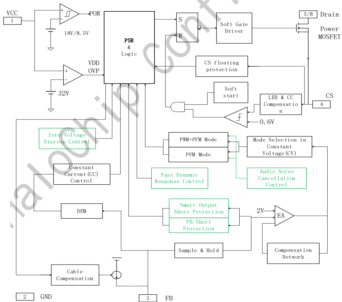
图 3 GP8642X 内部框图
