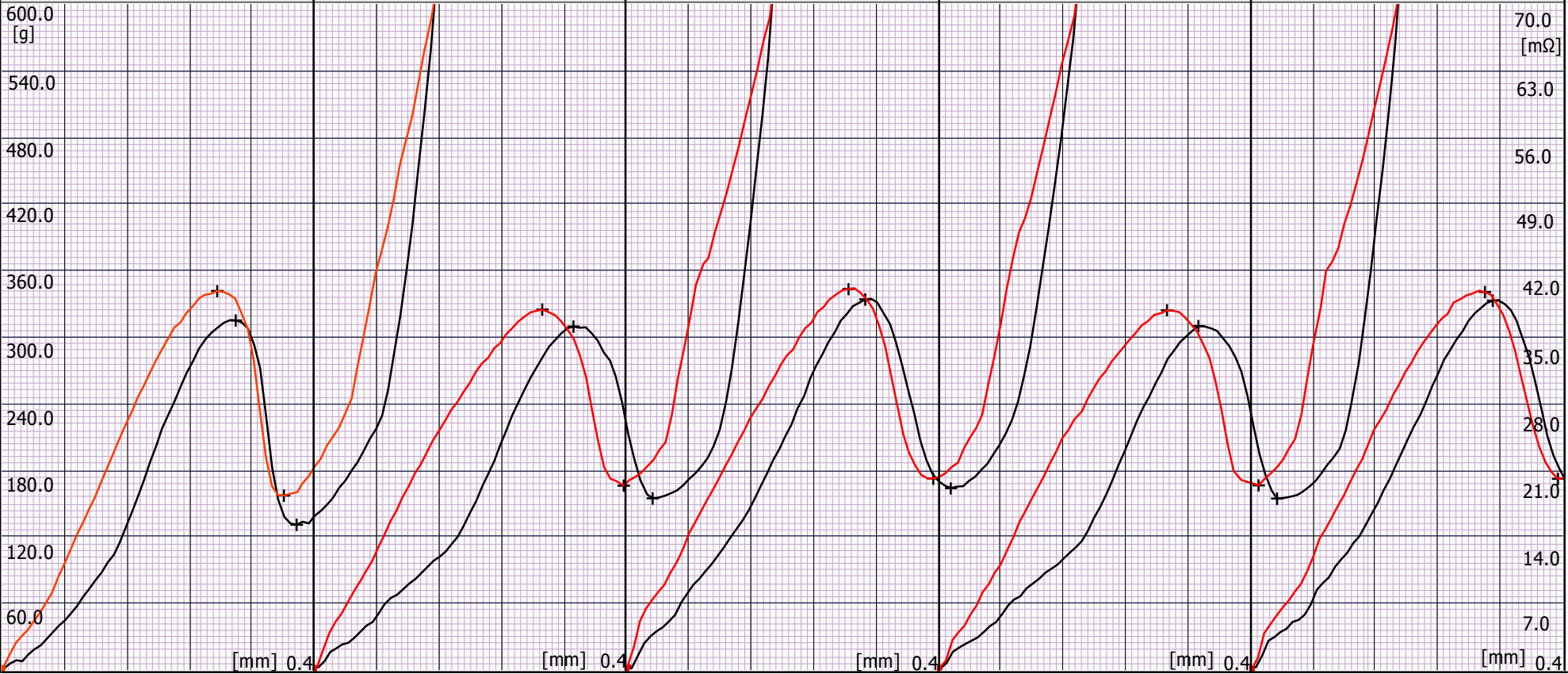
开关（荷重-行程）曲线测试图
