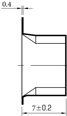
A-A剖面
