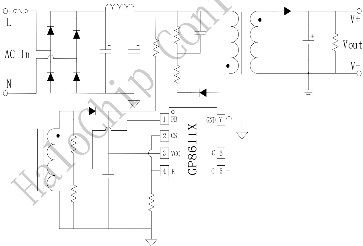
图 1 GP8611X 典型应用图
