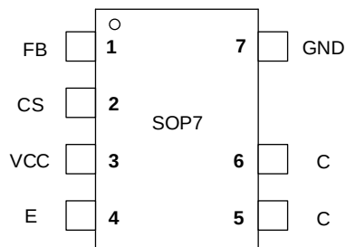
图 2 管脚封装图
