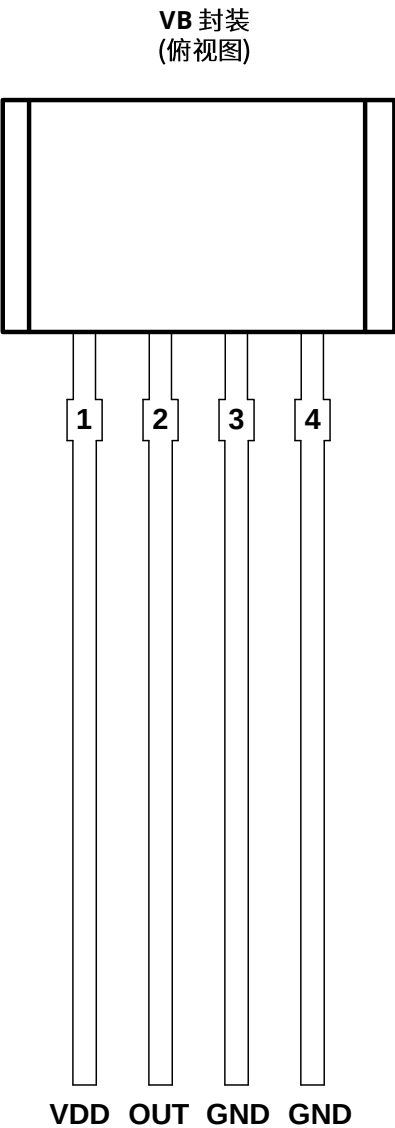
图 2 引脚描述
