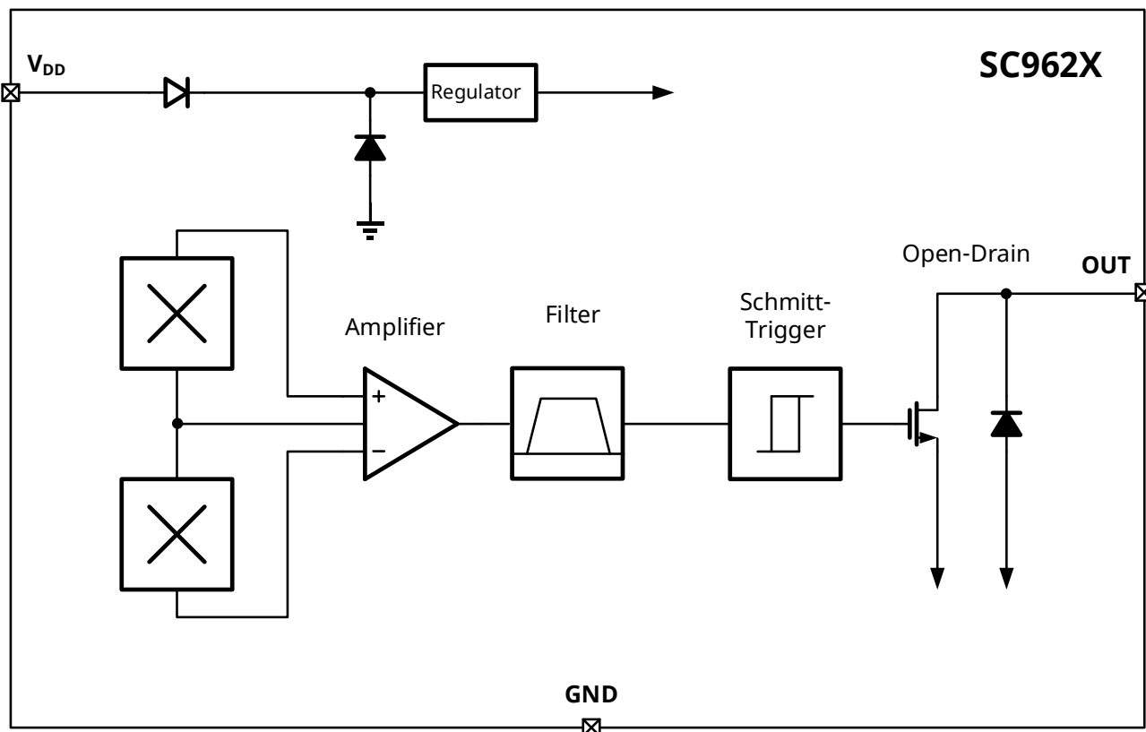
图 5 功能框图
