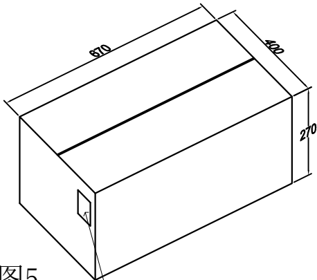
图5 外箱贴标处
