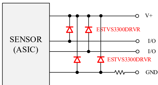
图 8 4 线制传感器应用
