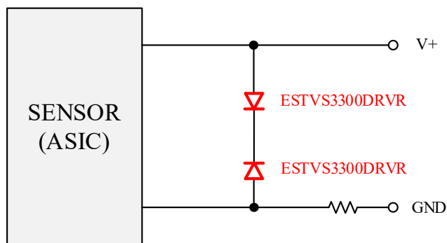
图 6 2 线制传感器应用
