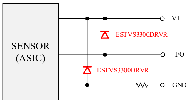
图 7 3 线制传感器应用
