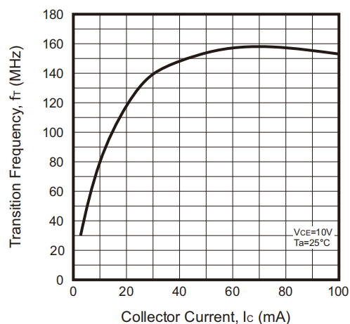
Fig.5 - f_T — I_C
