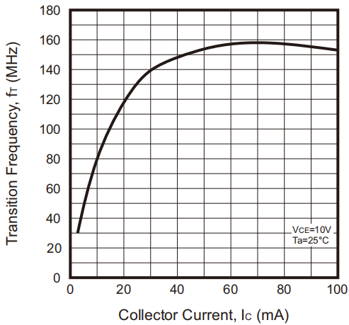
Fig.5 - f_T — I_C
