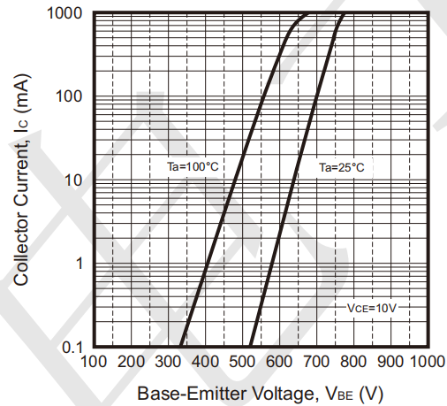
Fig.6 - I_C — V_{BE}
