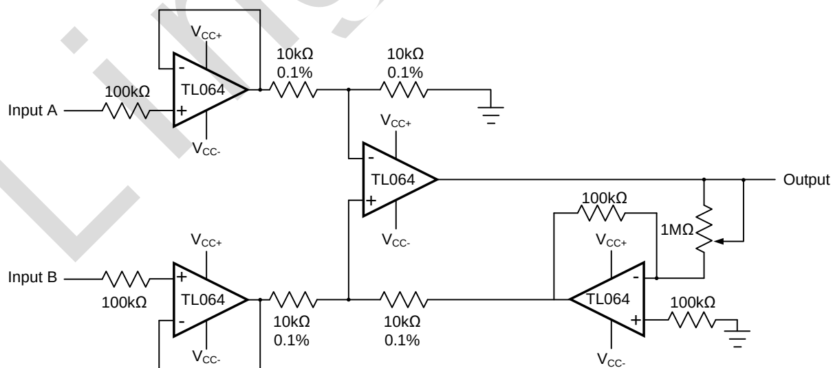
仪表放大器
