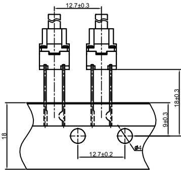
图1 编带图
