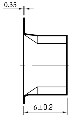
A-A剖面
