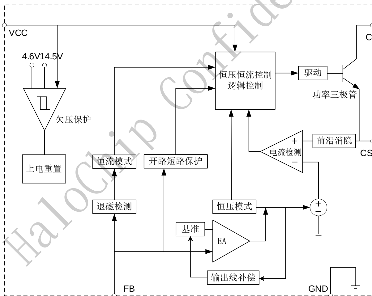
图 3 GP8672X 内部框图
