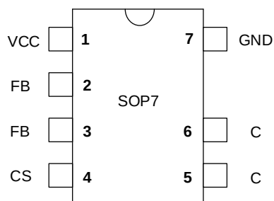
图 2 管脚封装图
