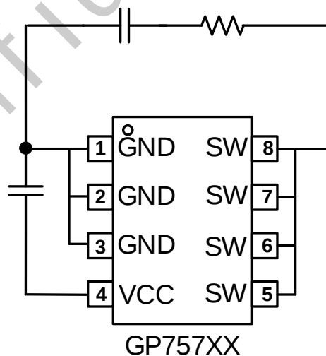
图 5 RC 吸收电路图
