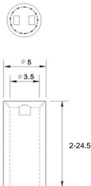
尺寸图
