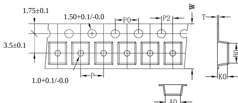
(1) 载带尺寸 (单位: mm)
