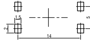
P.C.B. LAYOUT
