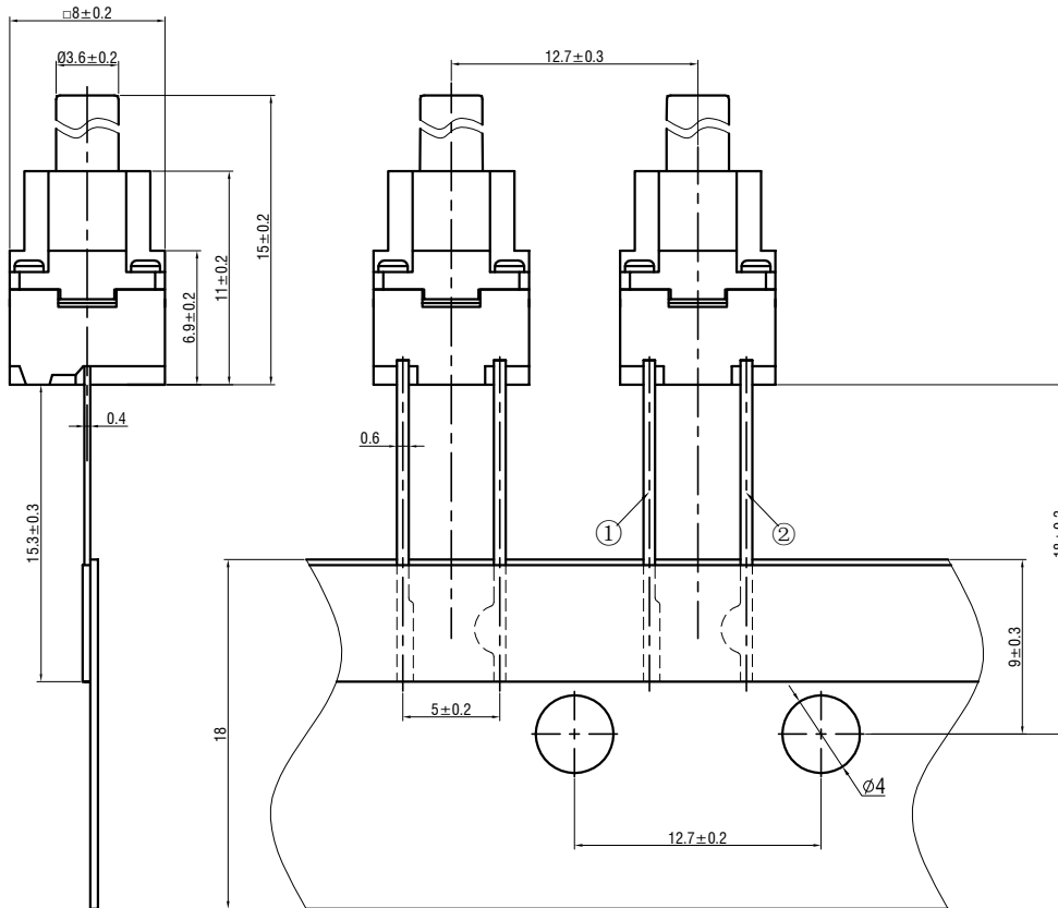
P.C.B. LAYOUT
