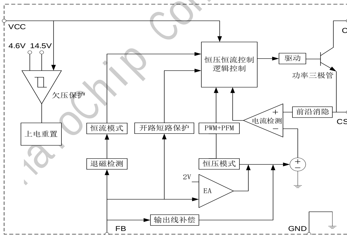
图 3 GP8655SX 内部框图
