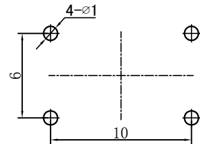
P. C. B. LAYOUT
