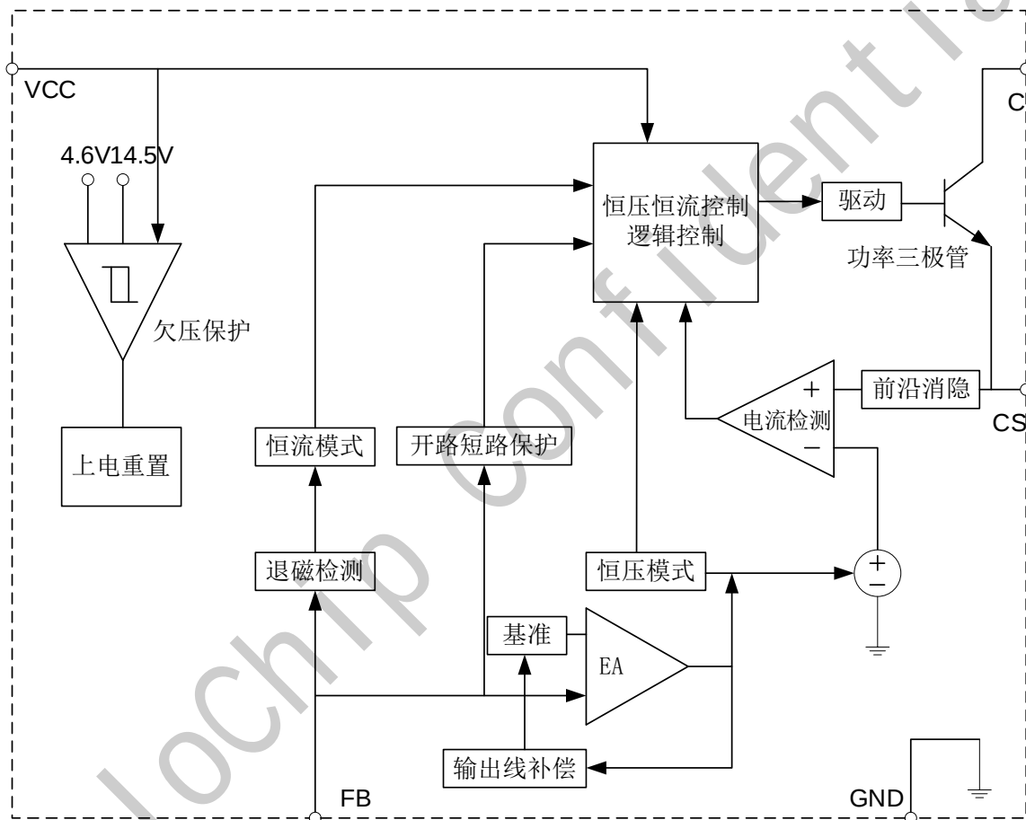
图 3 GP8615X 内部框图
