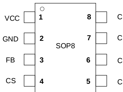
图 2 管脚封装图
