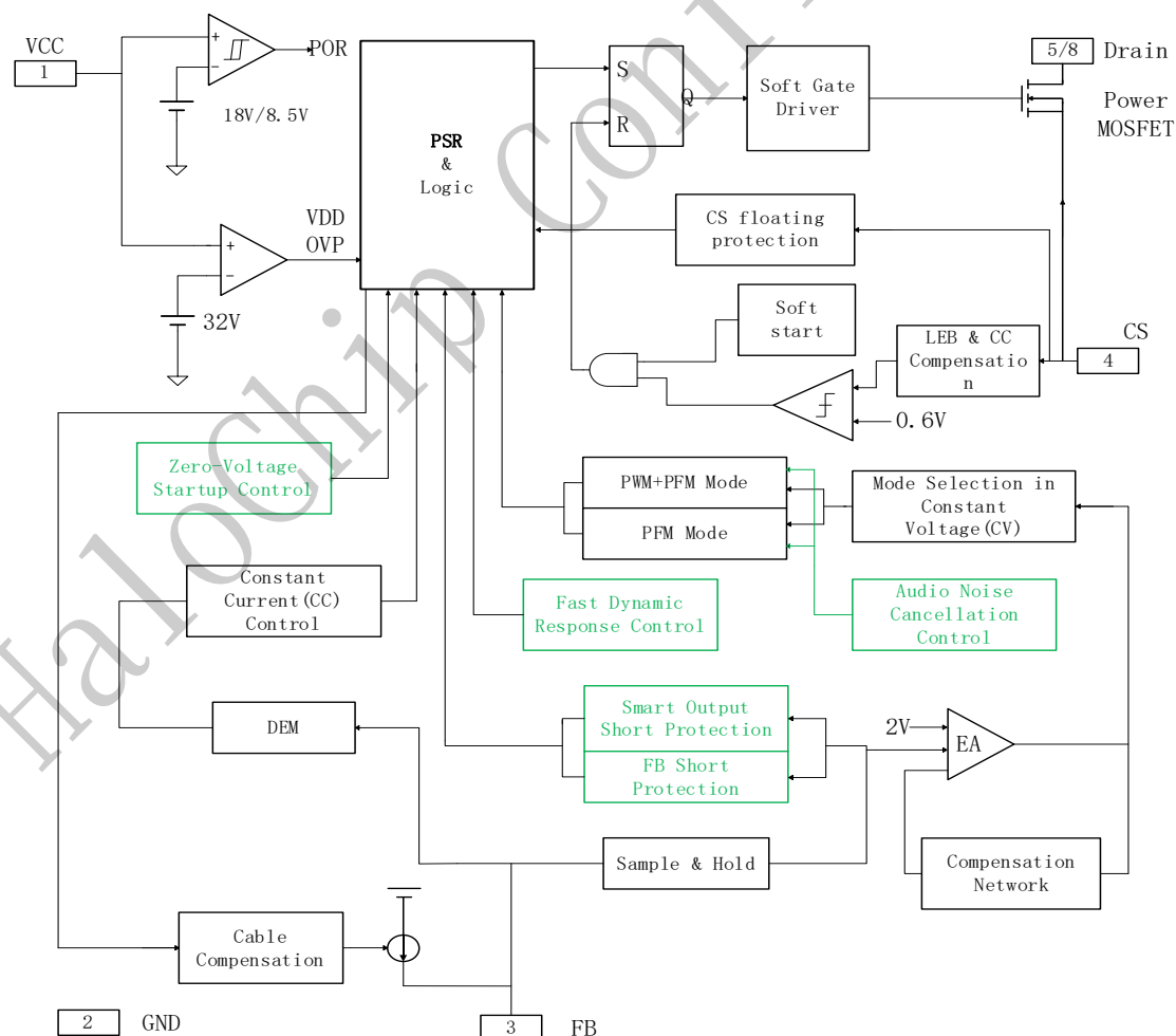
图 3 GP8682X 内部框图
