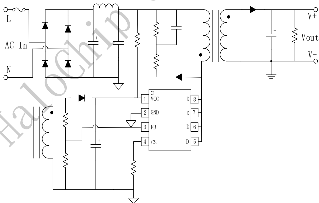
图 1 GP8682X 典型应用电路
