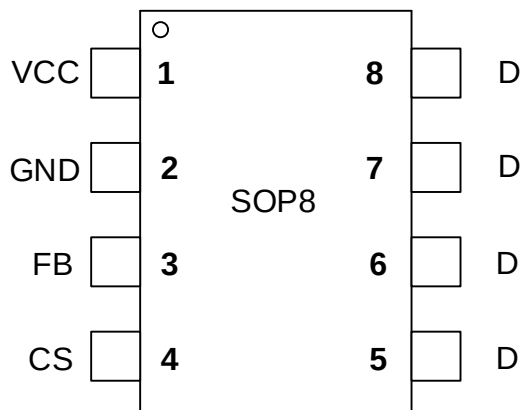
图 2 管脚封装图
