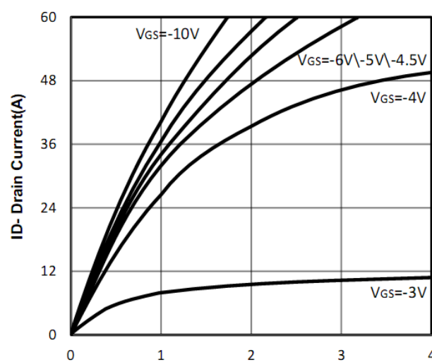
Figure4: -V DS -Drain-Source Voltage (V)
