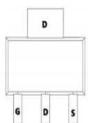
SOT89-3
