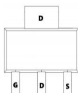
SOT89-3
