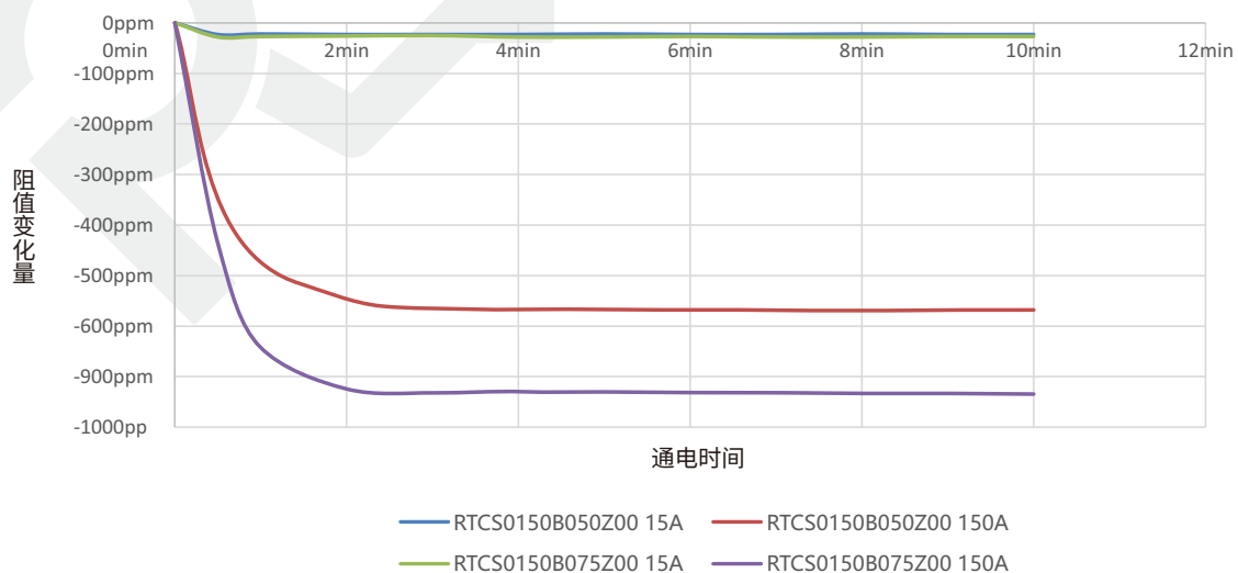
RTCS0150系列分流器通电电阻值变化情况
