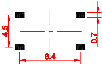
PCB. 焊接图
