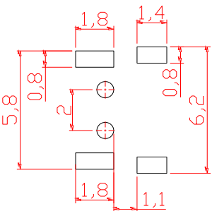
PCB 焊接图
