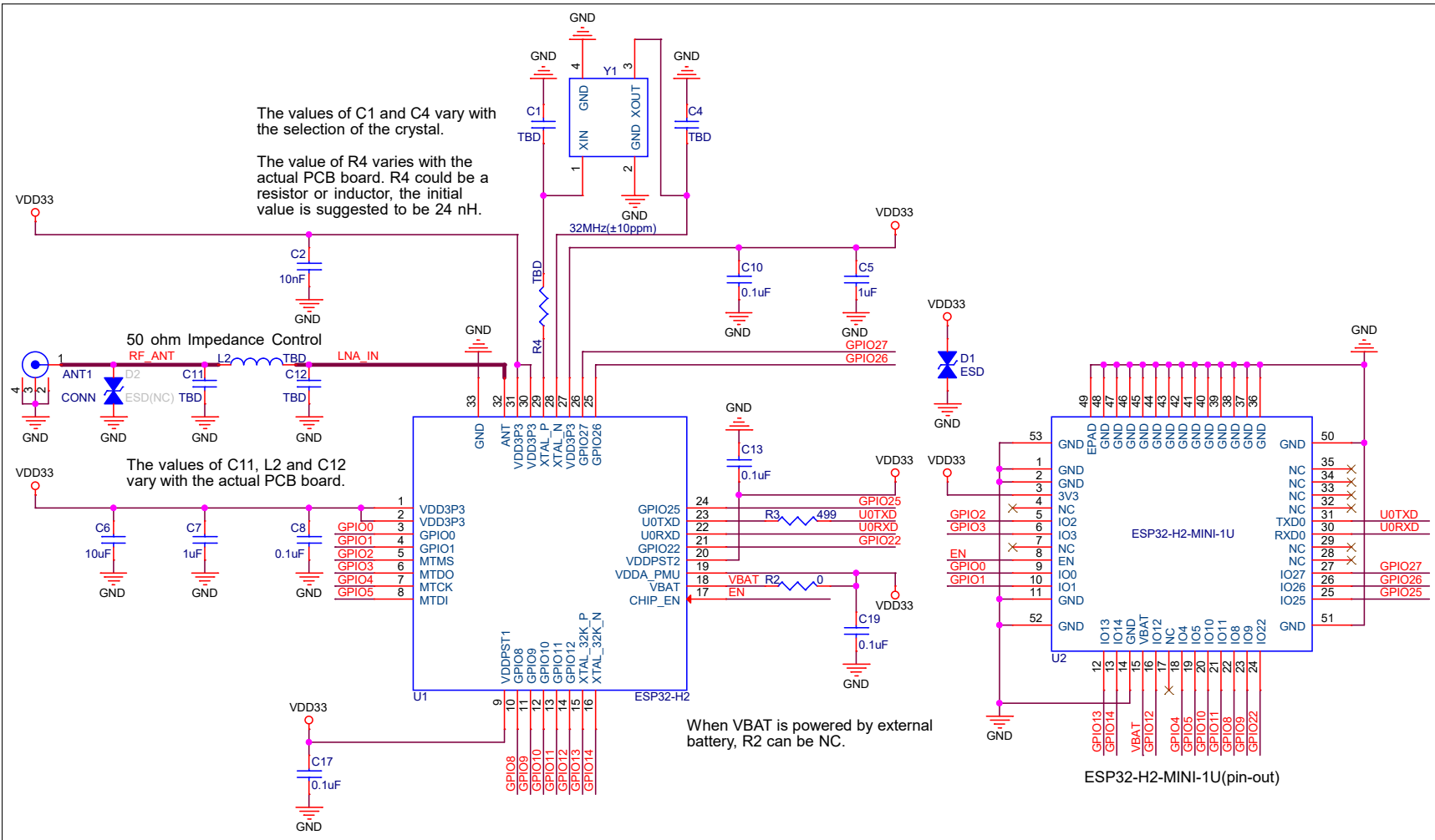
图 6: ESP32-H2-MINI-1U 原理图
