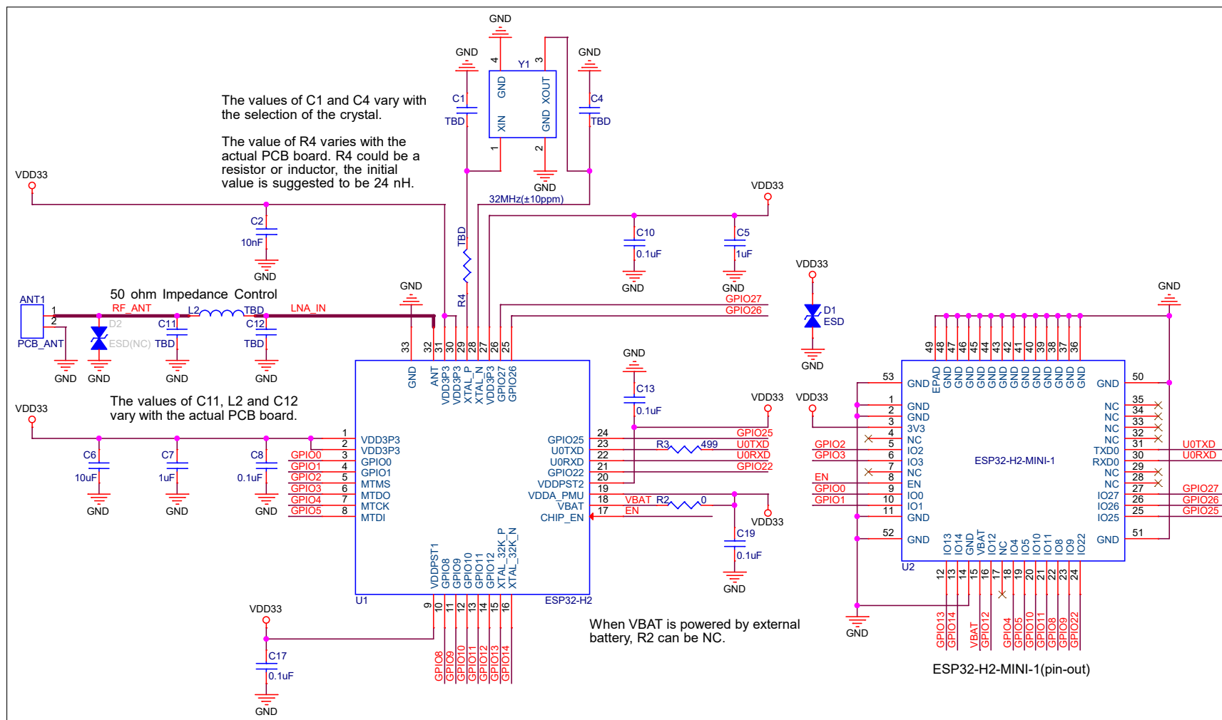
图 5: ESP32-H2-MINI-1 原理图
