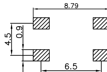
安装参考图
