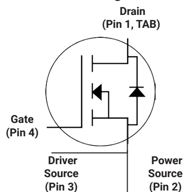
TO-247-4
