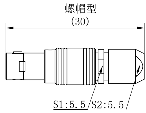
视图A
