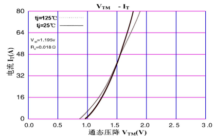
4、通态伏安特性曲线
