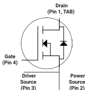
TO-247-4
